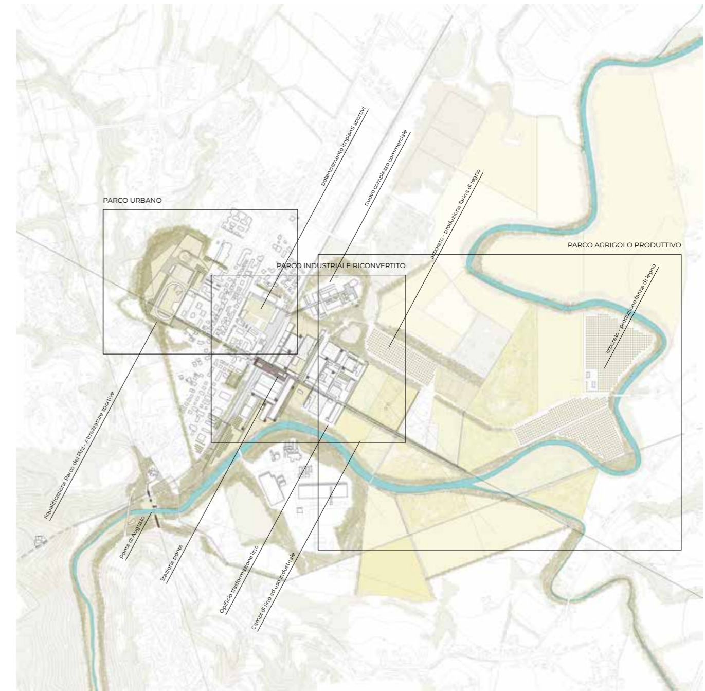
Planimetria generale.
