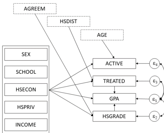
Figura 1: Path diagram di rappresentazione del modello. I tre riquadri in alto rappresentano le variabili strumentali. Le frecce con una singola direzione significano “spiega”. Le frecce a due direzioni indicano correlazione.
