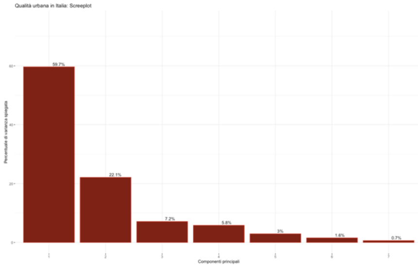
Figura 2: Analisi in componenti principali - percentuale di varianza spiegata da ciascuna componente
