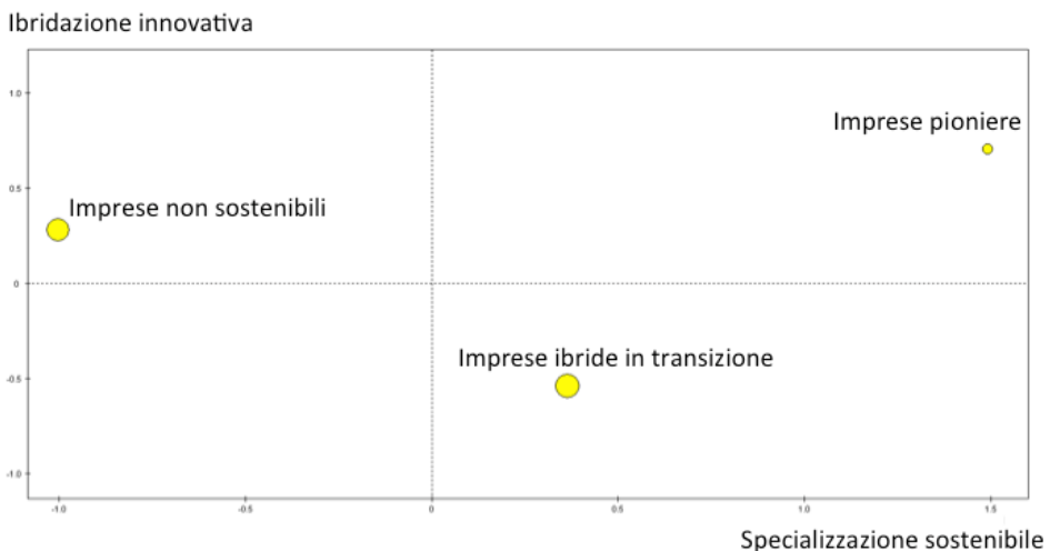
Figura 1: Proiezione dei cluster sui primi due fattori estratti dall'acm
