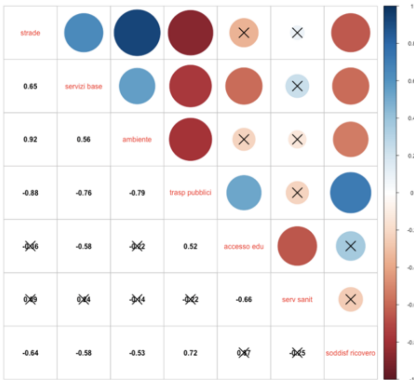
Figura 1: grafico delle correlazioni tra le sette dimensioni considerate. Sotto la diagonale principale è riportato il valore numerico delle correlazioni e sopra lo stesso rappresentato graficamente
