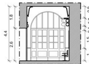
Sezione CC
