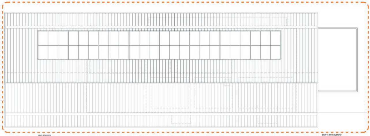
PIANTA COPERTURE
