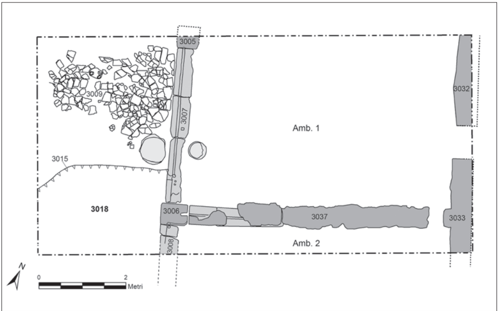
Fig. 4 – Planimetria delle strutture rinvenute nel saggio 3 con indicazione delle principali US menzionate nel testo (dis. S. De Togni).
