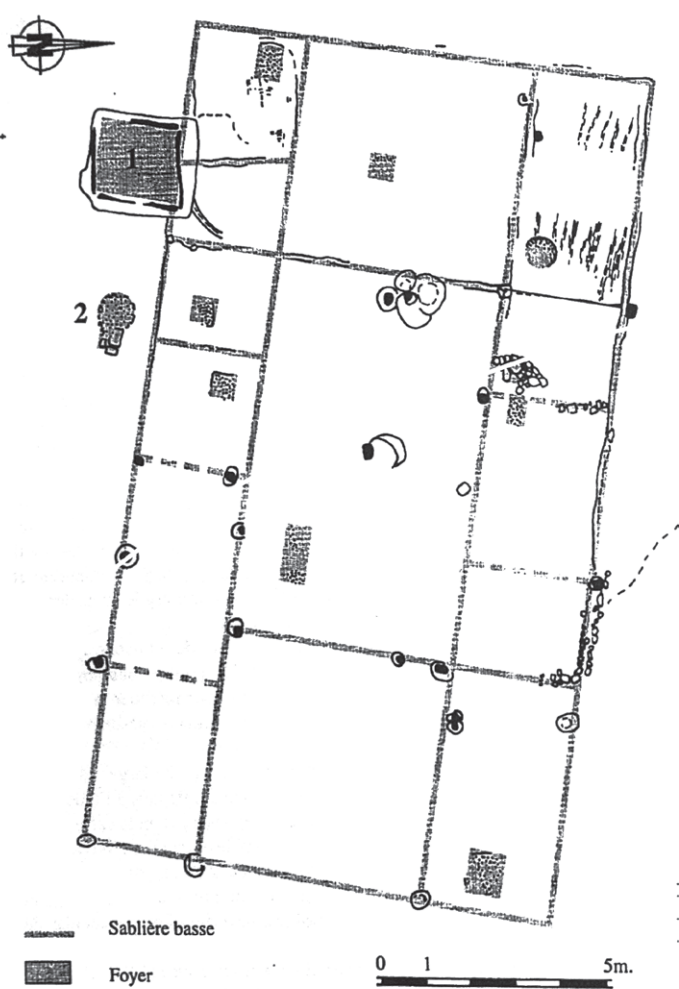
Fig. 4 Hamage, planimetria dell'edificio ligneo della fase IIIA (da Louis 1997)
