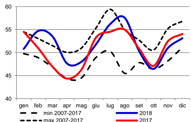
Figura 4.31 - Punta di domanda in potenza mensile (GW)
