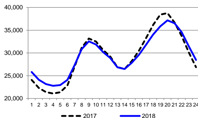
Figura 4.36 Profilo orario della domanda totale e della domanda residua – Sistema Italia (MW)
