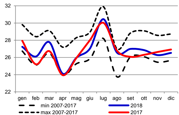
Figura 4.30 - Richiesta di energia elettrica mensile, dati storici "depurati" e trend di lungo periodo (GWh)
