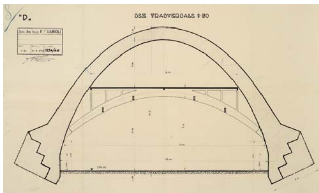
Fig. 3. Disegno di sezione dell'aviorimessa di Pantelleria, 1937. Progetto della Società Anonima Fratelli Ingg. Damoli (Archivio Storico dell'Aeronautica Militare, Roma).
