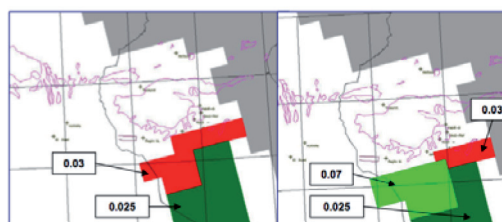
Fig. 2b - Adattamento della distribuzione del coefficiente di immagazzinamento - Storage coefficient distribution adjustment
