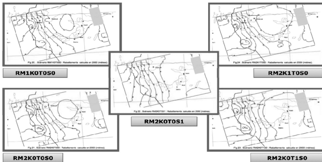
Fig. 7 - Abbassamenti stimati dal modello NDRM al 2050 - Drawdown estimated by NDRM model at 2050
