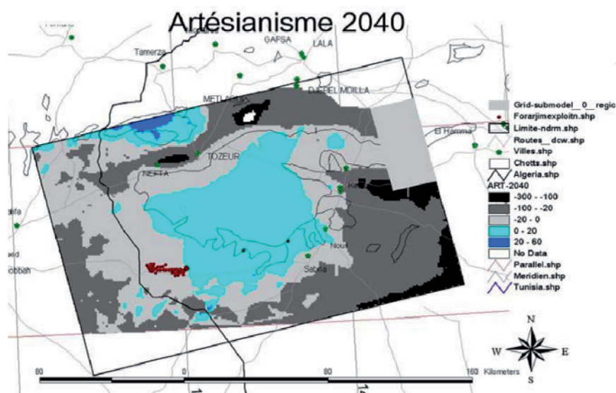
Fig. 8 - Distribuzione dell'artesianismo residuo al 2040 per lo scenario RM1K0T0S0 - Artesianism amount at 2040 for the RM-1K0T0S0 scenario
