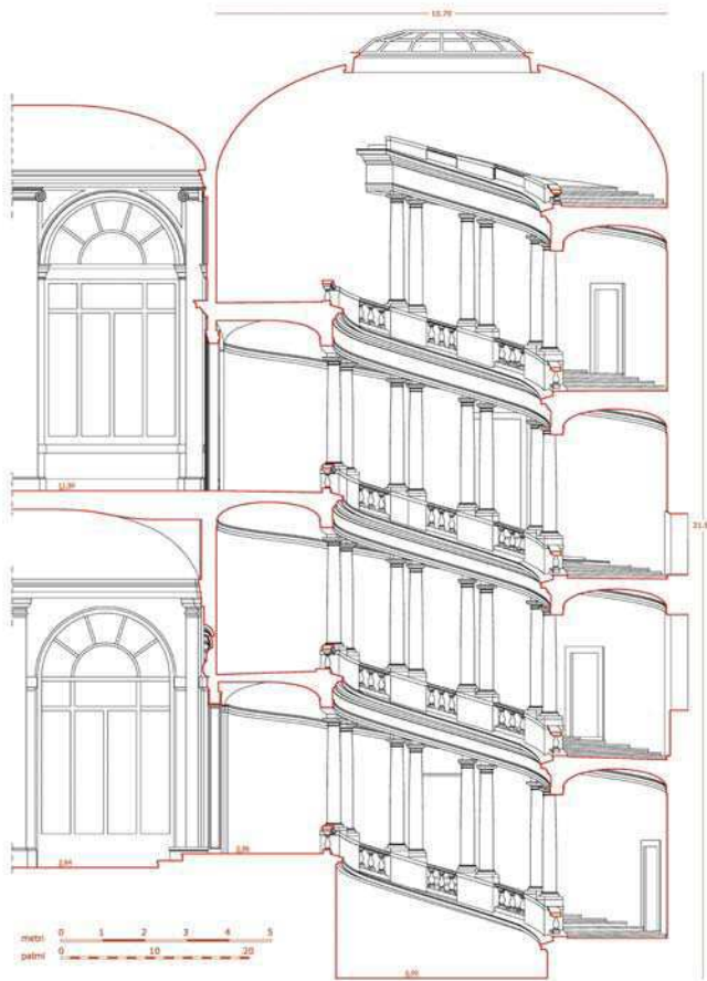
Fig. 2. Roma, palazzo del Quirinale, sezione centrale sul lato maggiore della scala ovale (rilievo di Leonardo Paris).
