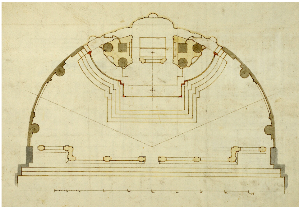
fig. 117: Carlo Fontana, progetto per altare e cripta per la chiesa del Gesù, Stoccolma, Nationalmuseum, CC 878 v.
