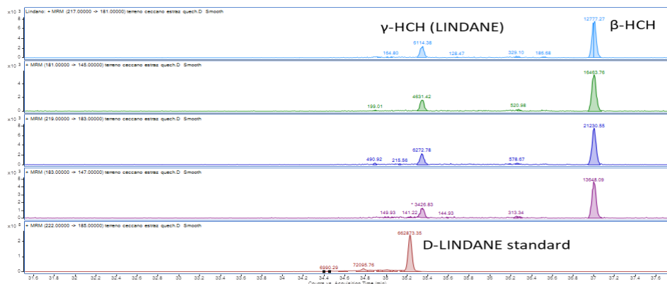
Figura 2: Cromatogramma
