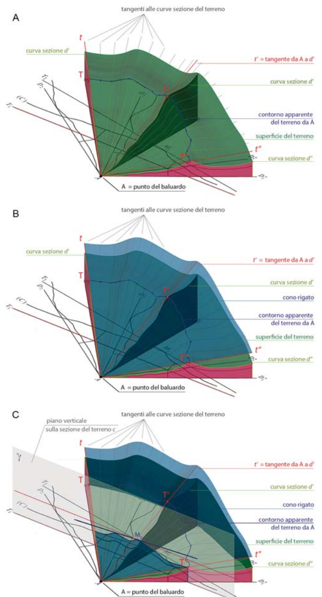
Fig. 1. Studio del défilement : metodo proposto da Monge suddiviso in fasi.
