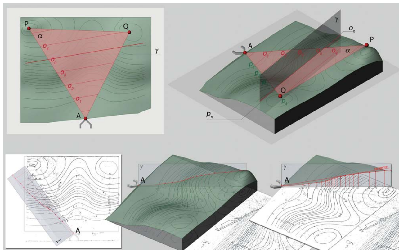
Fig. 2. Studio del défilement di una fortificazione. In alto: metodo proposto da A.-N.-B. du Vignau; in basso: metodo proposto da J.-B. Meusnier de la Place.
