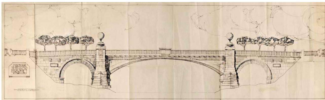
Fig. 3. G. Giovannoni, progetto del Ponte Tito Tazio, città giardino Aniene. (Roma, Archivio del Centro di Studi per la Storia dell'Architettura).
