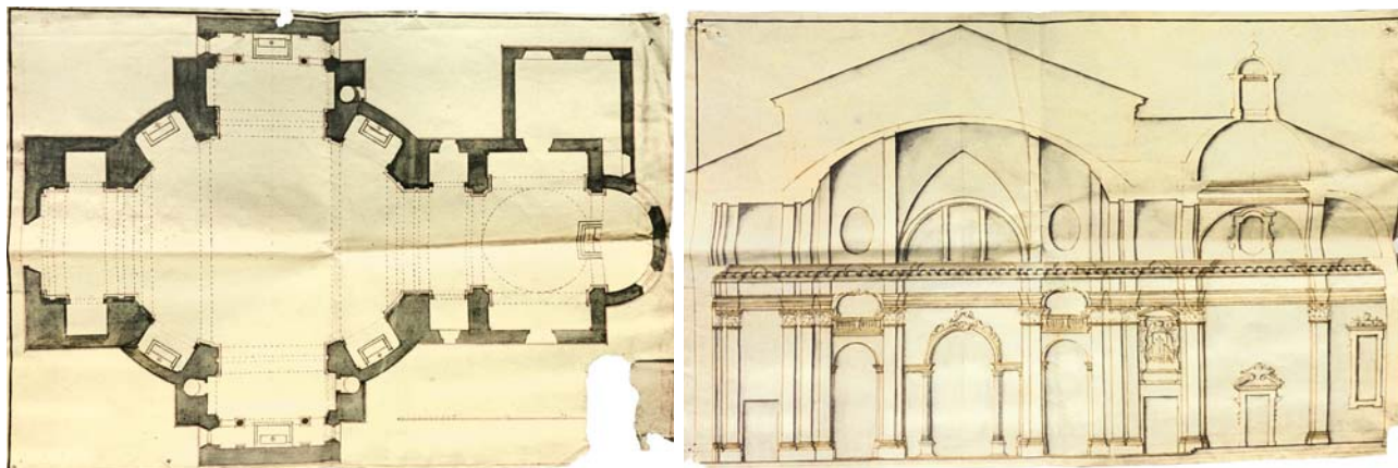
Fig. 2. Chiesa di San Giovanni Battista a Morbegno, pianta e sezione longitudinale del progetto seicentesco. (Archivio dell'Annunziata di Como).
