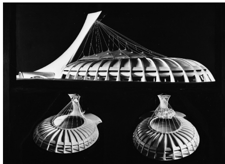
[Fig.3] Modello dello Stadio Olimpico 11 aprile 1972. © Ville de Montréal Id.CA M001 VM094 Y-1-10-D022
