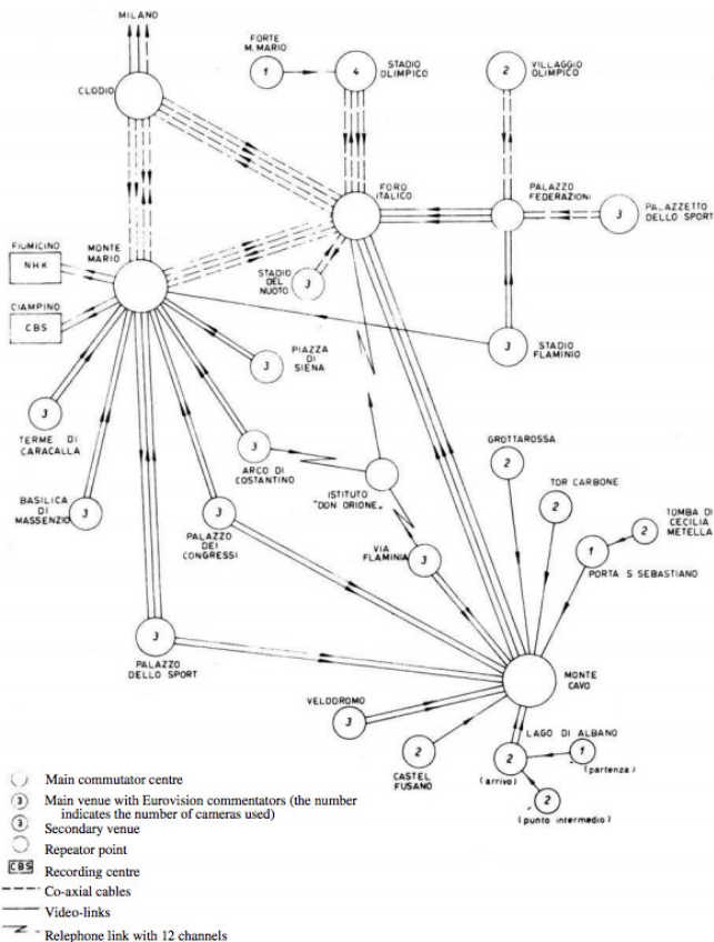
[Fig.18] VIDEO-LINK NETWORK rete di trasmissione televisiva geografia di connessione tra i differenti siti dell'evento, in CIO(1960) Rome Olympic Games Official Report Volume One - Description , p.386
