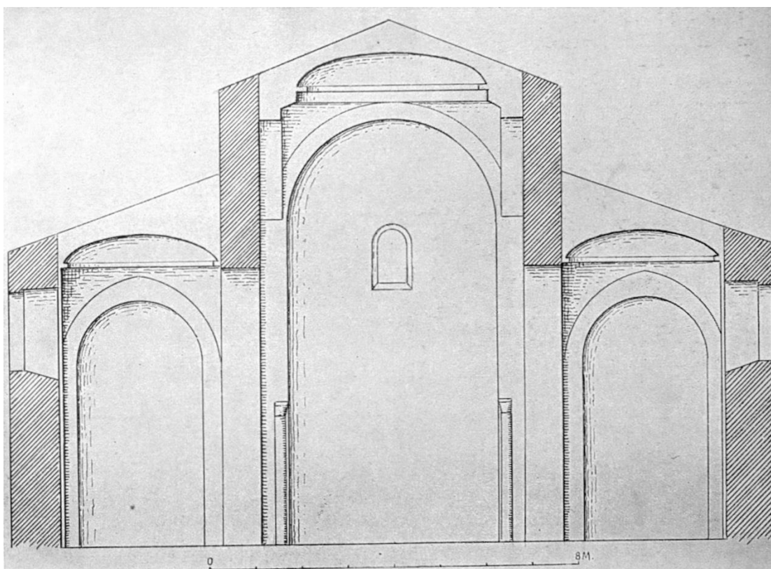
2. Sezione trasversale delle absidi (da ORSI 1929)
