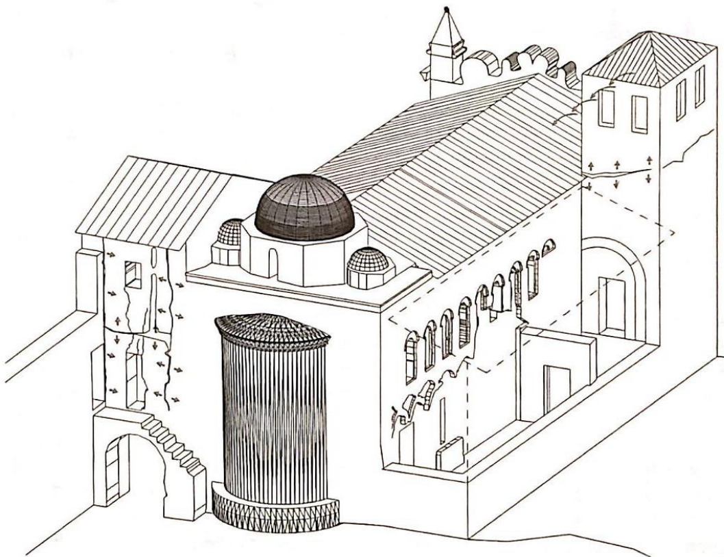
2. Assonometria con schema dei fenomeni di collasso in corso (da TODESCO 2007)
