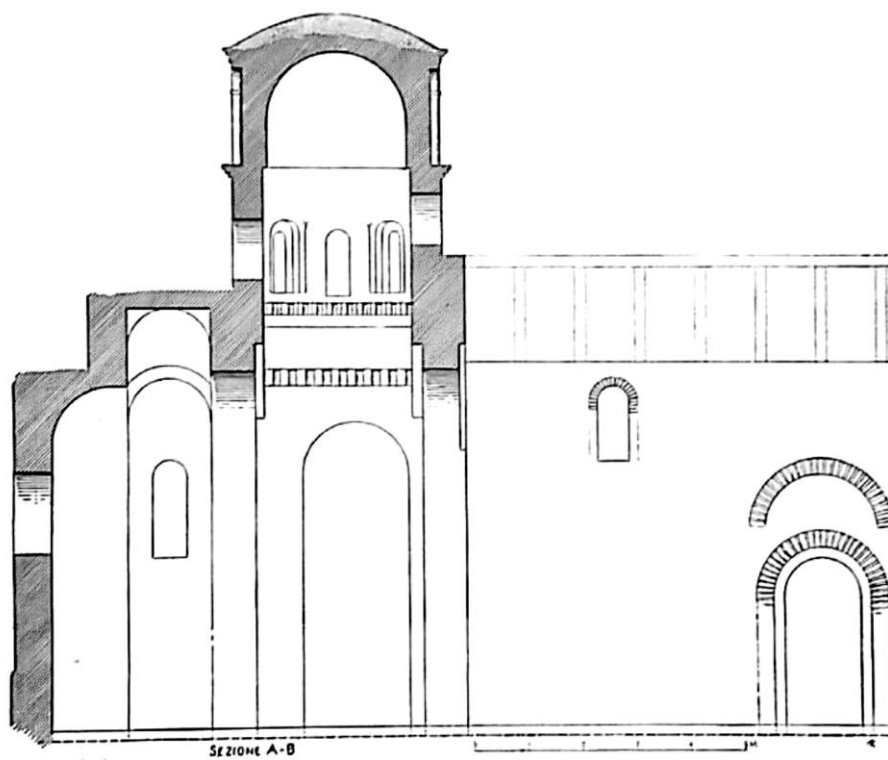
2. Spaccato longitudinale (da ORSI 1929)
