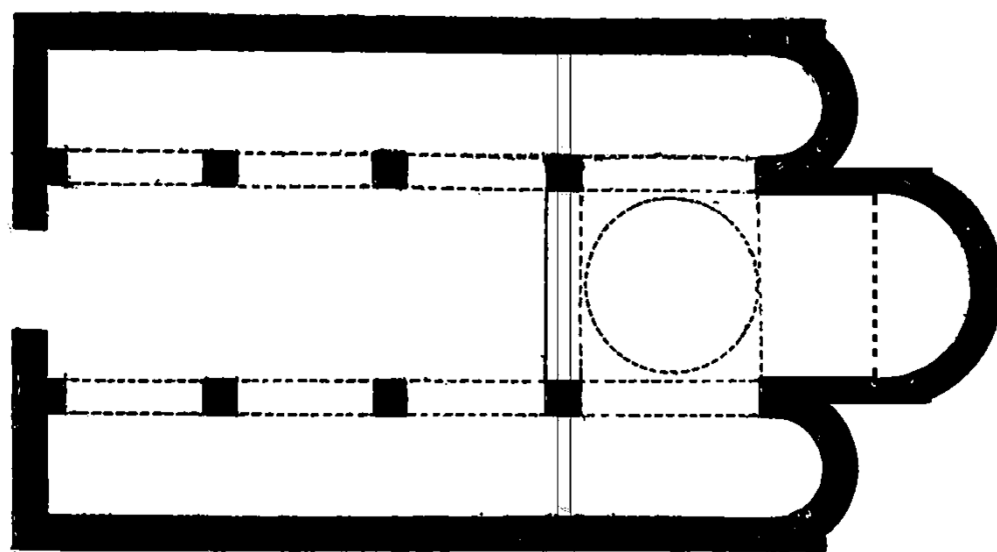
2. Pianta restitutiva aggiornata in base alla perizia del 1840
