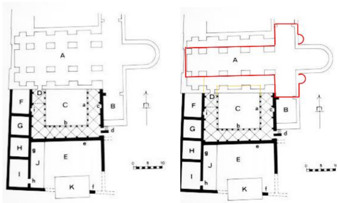
1-2. Pianta del complesso cattedrale attuale (da BERNABÒ BREA 1988). A: cattedrale; B: cappella del SS. Sacramento; C: chiosstro; D: battistero; E: cortile epigrafico del museo; F, G, H, I: sale del museo; K: padiglione epigrafico. A destra ipotesi restitutiva della pianta originale
