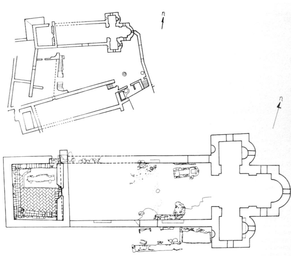
1. Pianta del complesso abbaziale e dei ritrovamenti nell'area della chiesa degli scavi del 1990 (da IANNELLI 2000)
