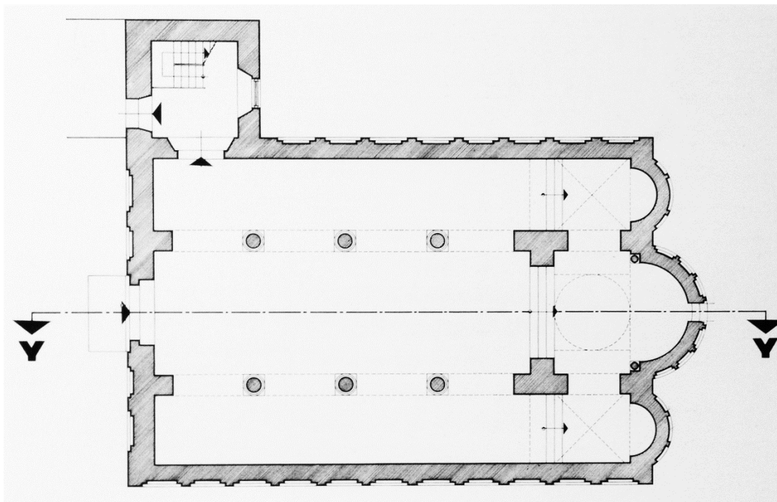
1. Pianta (da CIOTTA 1976)
