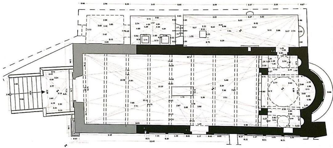
1. Pianta (da TODESCO 2007). In nero le porzioni murarie medievali
