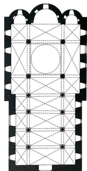
46. Messina, Badiazza, pianta (da BELLAFFIORE 1993)
