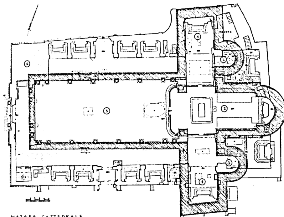
MAZARA CATTEDRALE Pianta. Consistenza attuale con lo schema dell'impianto ruggeriano. 1 Prothesis 2 Bema 3 Diaconicon 4 Transetto 5 Asila 6 Torre campanaria del 1654
