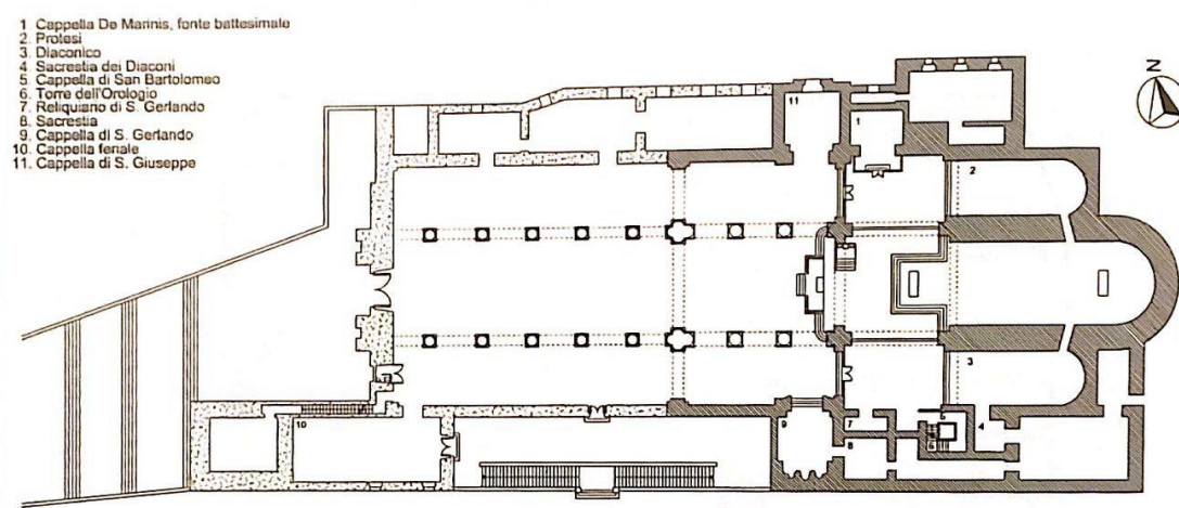
3. Pianta secondo SCHMIDT 2010
