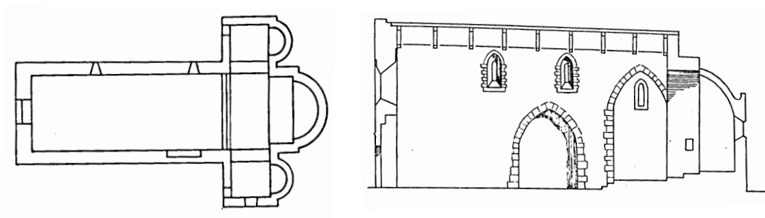
1. Pianta e sezione longitudinale (da SCHWARZ 1942-1944)
