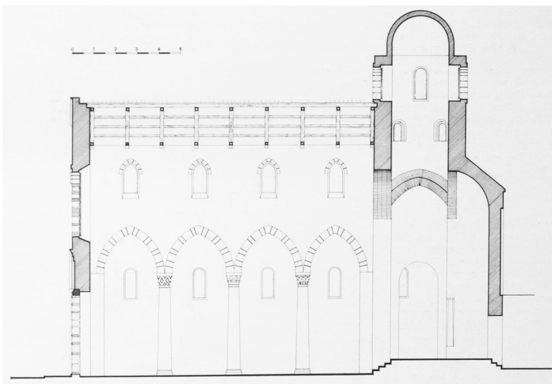
2. Sezione longitudinale (da CIOTTA 1976)
