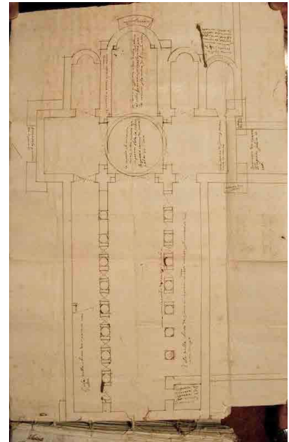
2. ACGR, vol. 85, tav. f. t., rilievo dei danni del sisma del 1638 (da ROMEO 2014-2015)
