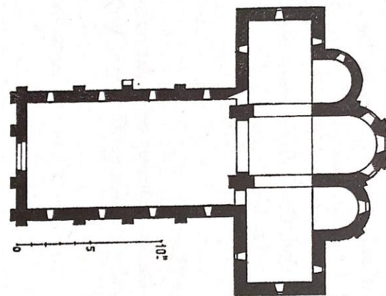
20. Meusnes (Loir-et-Cher), Saint-Pierre, pianta (da KONERDING 1976)
