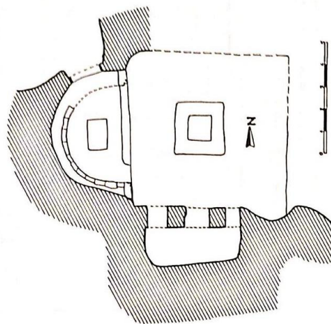
5. Pianta della chiesa semi-ipogea (da GIGLIO 2002)
