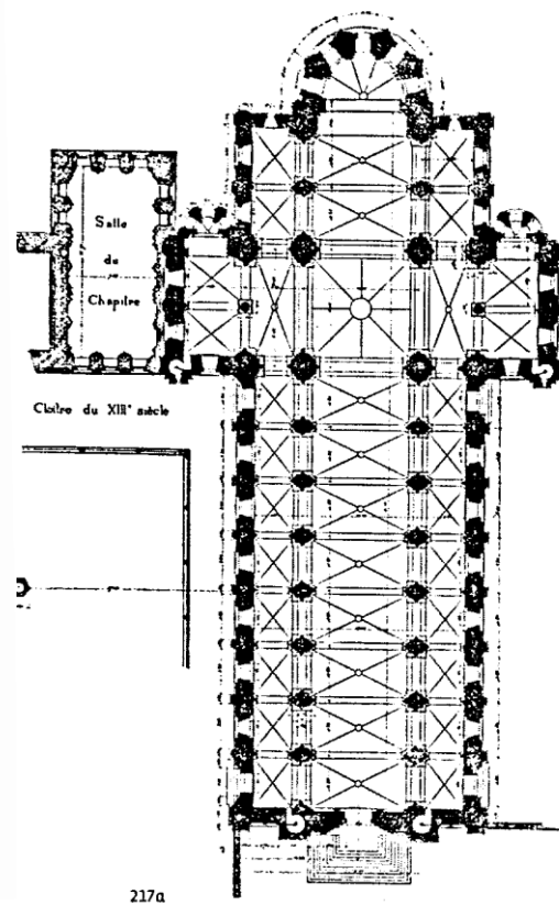
6. Saint-Martin de Boscherville (Seine-Maritime), Saint-Georges, pianta (da CHAIX 2011)
