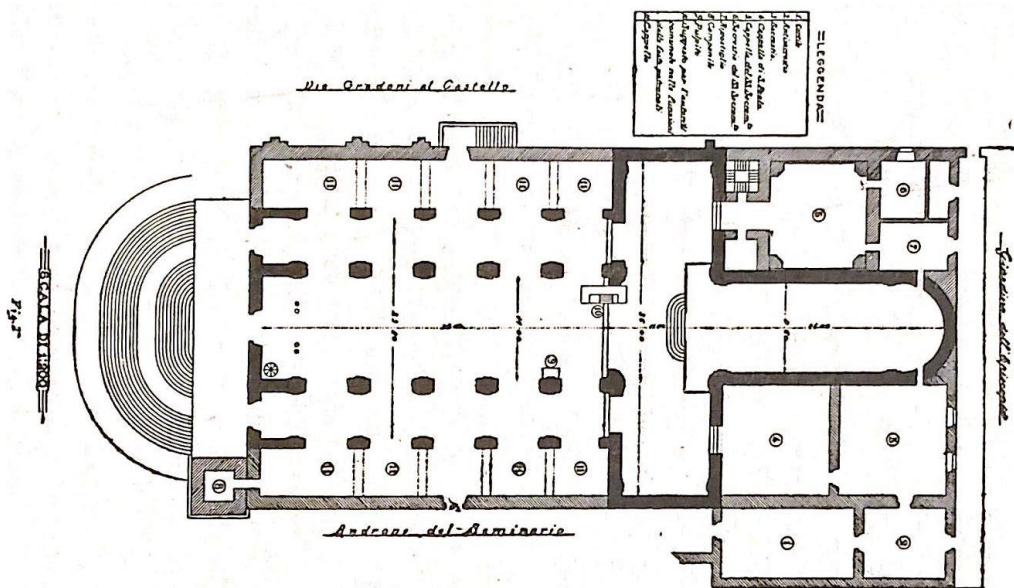
2. Pianta della cattedrale ante 1908, in nero le parti riferite all'età normanna (da DE NAVA 1941)
