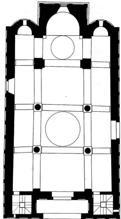
48. Casalvecchio Siculo, Ss. Pietro e Paolo d'Agrò, pianta (da BELLAFIGLIO 1990)
