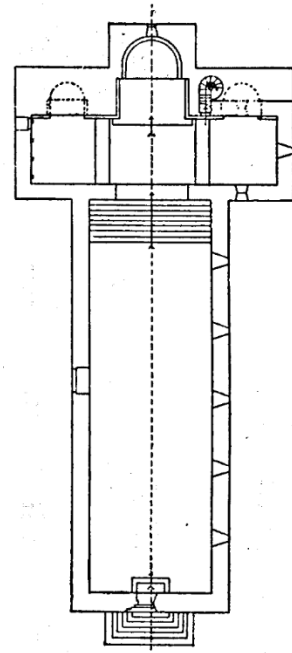
18. Piazza Armerina, S. Andrea del Priorato, pianta (da BELLA 2012)
