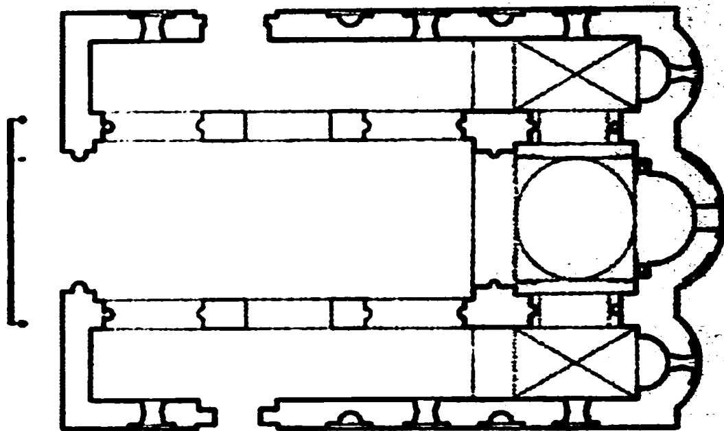
1. Pianta (da BOZZONI 1999)
