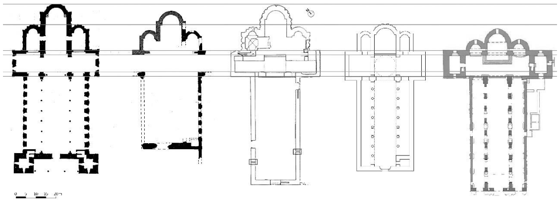
1. Planimetrie a confronto di (a partire da sinistra): cattedrale di Cefalù, S. Maria di Sant'Eufemia, S. Maria della Roccella, SS. Trinità di Mileto, cattedrale di Catania.
