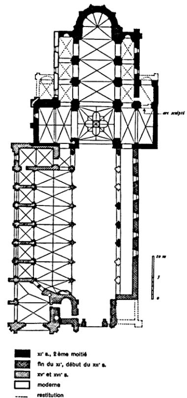
8. Montivilliers (Seine-Maritime), Notre-Dame, pianta (da CHAIX 2011)
