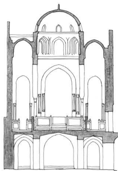
70. Palermo, Cappella Palatina, sezione trasversale (da DI STEFANO 1955)
