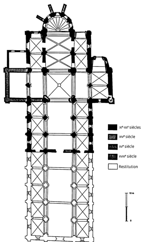
7. Cerisy-la-Forêt (Manche), Saint-Vigor, pianta (da CHAIX 2011)
