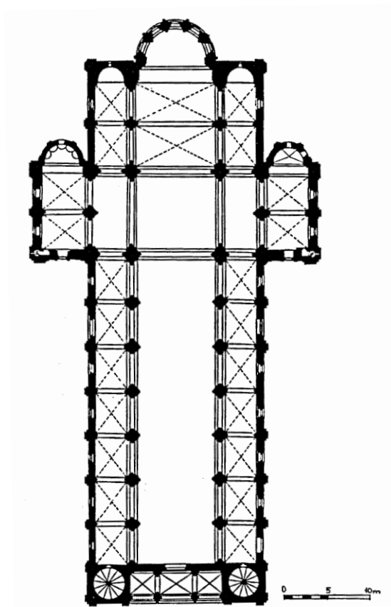
5. Caen (Calvados), Saint-Nicolas, pianta (da CHAIX 2011)
