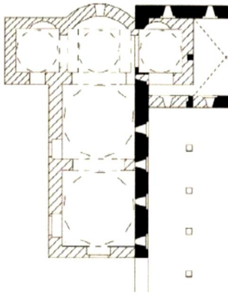
17. Palermo, S. Giovanni degli Eremiti, pianta (da BELLAFFIORE 1990)
