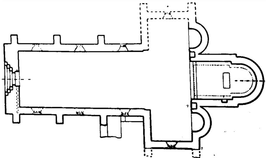
1. Pianta (da DI STEFANO 1955)
