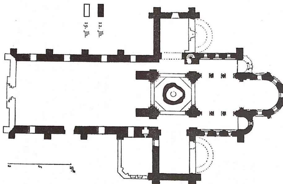
22. Les Aix-d'Angillon (Cher), Saint-Germain, pianta (da KONERDING 1976)
