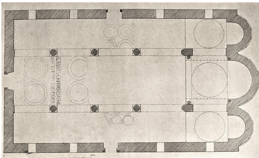
1. Pianta con aggiunta delle arcate di imposta della cupola (rielaborazione da ORSI 1929)
