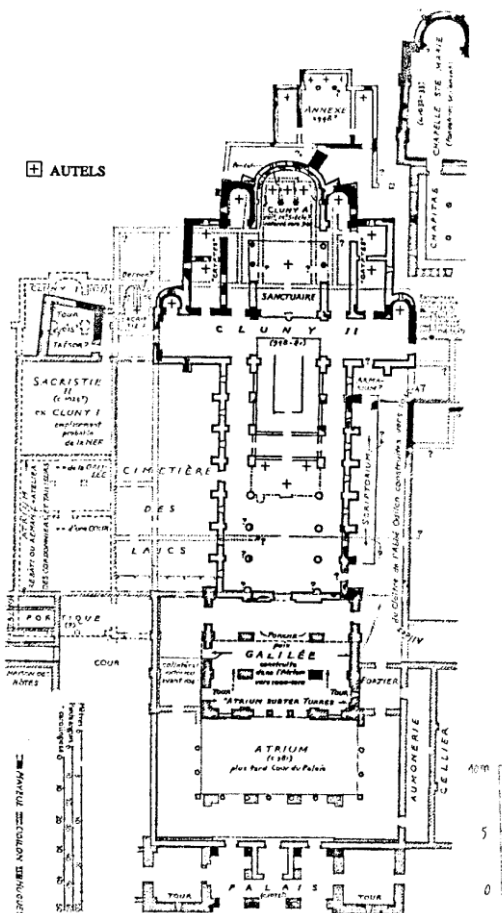
3. Cluny II, pianta (da CONANT 1968)
