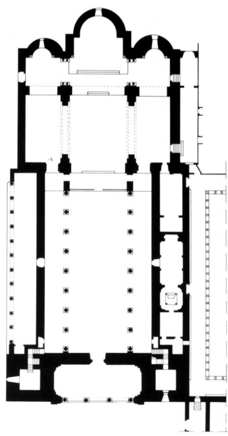
15. Monreale, cattedrale, pianta (da Bellafigliore 1990)
