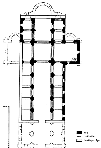
4. Bernay (Eure), Notre-Dame, pianta (da CHAIX 2011)
