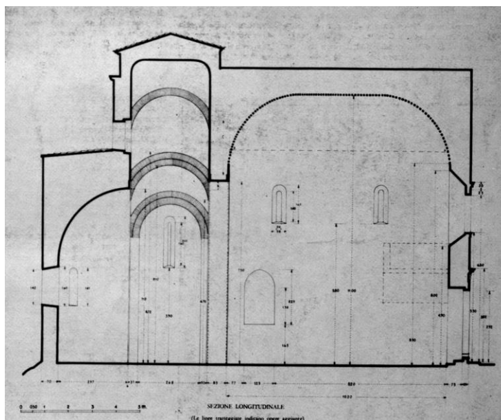
2. Sezione longitudinale (da CIOTTA 1976)
