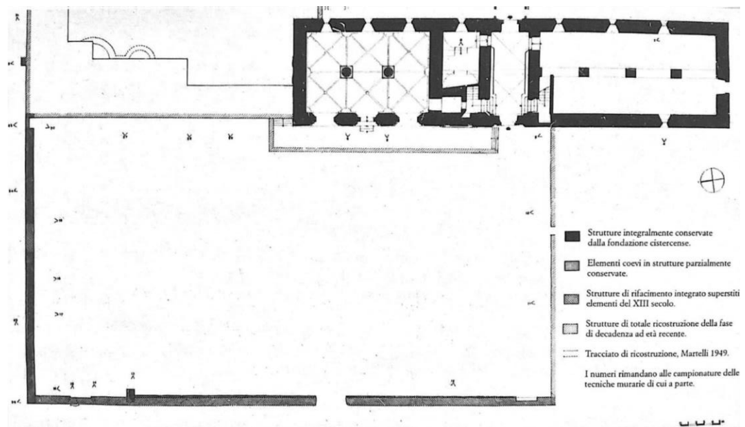
2. Rilievo dei resti dell'abbazia, stato attuale (da ZINZI 1999)
