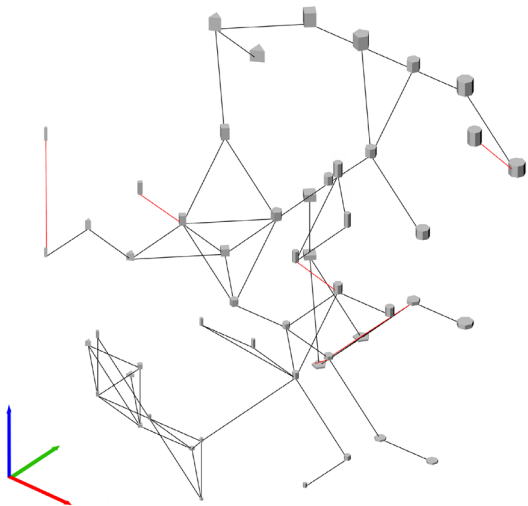
Fig. 11: Diagramma di Delaunay rappresentante la rete di connessioni all'interno del museo.
