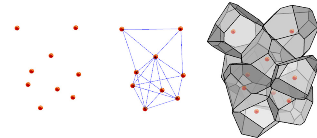
Fig. 7: Tetraedralizzazione di Delaunay e cellule di Voronoi generate da una serie finita di punti disposti nello spazio 3D. La rete di Delaunay corrisponde a tutti i possibili percorsi all'interno del museo.
