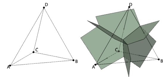
Fig. 6: Diagramma di Voronoi relativo a quattro punti nello spazio. I sei piani che suddividono lo spazio sono normali ai segmenti che connettono i punti e passano per il loro punto medio.
