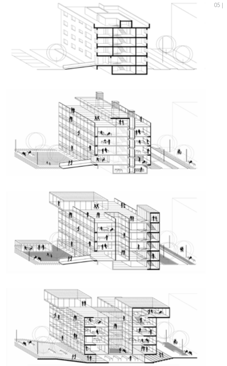
05 | Abaco degli interventi di Riqualificazione / Rigenerazione / Rinnovo sugli edifici oggetto della sperimentazione sul quartiere di Casale Caletto. Dall'alto al basso: Stato attuale, interventi di Soft retrofit, Medium retrofit e Hard retrofit Chart of activities comprising Retrofit / Regeneration / Renewal of buildings subject to experimentation in Casale Caletto neighbourhood. From top to bottom: Current state, soft retrofit, medium and hard retrofit
