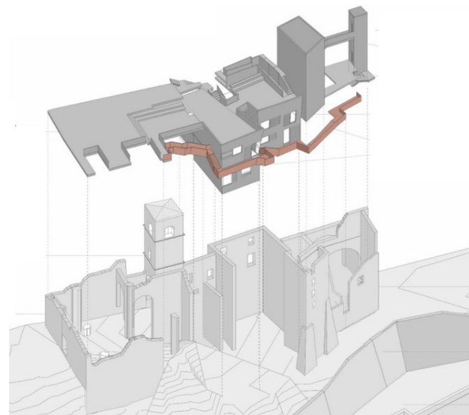
Fig 24. Inserimento nel nuovo progetto all'interno dell'edificio esistente. Elaborazione Simone Moneta
