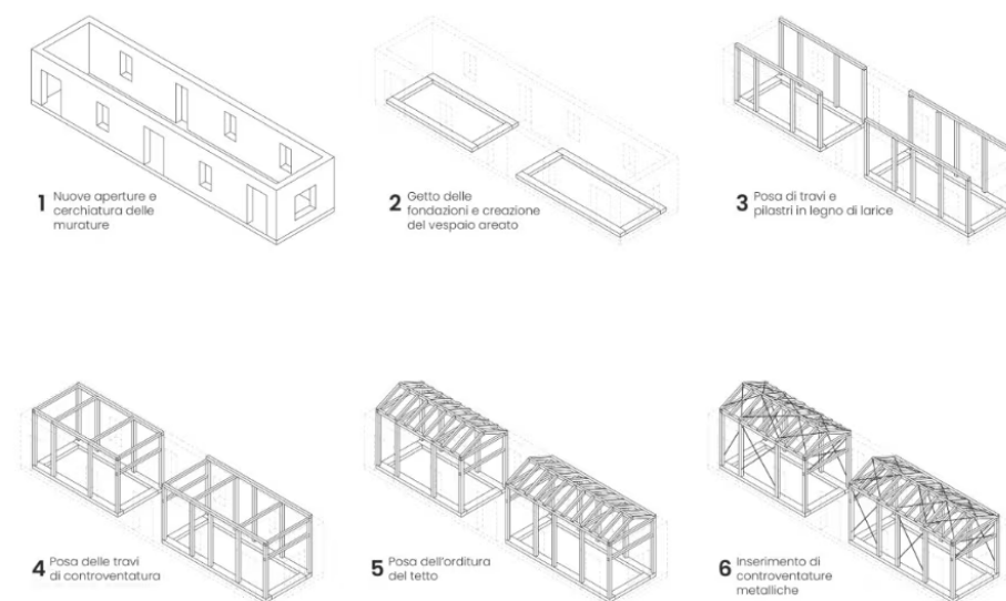
Fig. 24. Fasi costruttive. Foto rmedium
