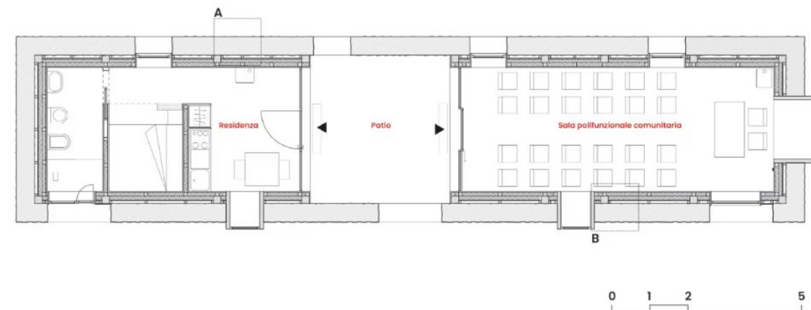
Fig. 26. Pianta Casermetta a sud. Foto rmedium
