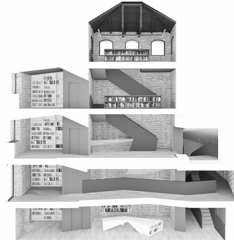
Fig. 28. Sezione della torre e dei due edifici adiacenti. Foto cn10architetti
