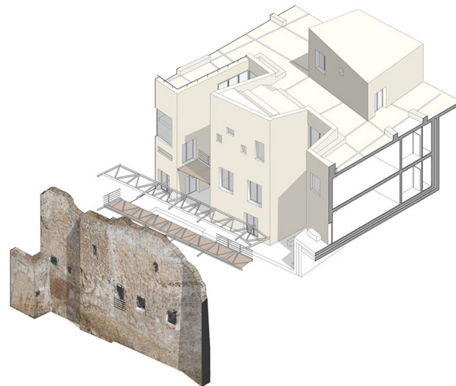
Fig 30. In alto modello del nuovo edificio dietro le mura esistenti, consolidate attraverso una passerella pedonale che permette l'ancoraggio delle stesse alla nuova struttura.
