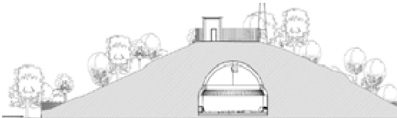
Fig. 216 – Sezione trasversale sulla parte terminale della camera sepolcrale estratta dal modello informato del Mausoleo di Monte del Grano.
