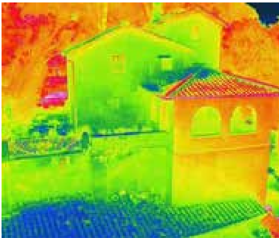
Fig. 169 – Immagine termografica della facciata esterna rivolta a nord del complesso del Sepolcro degli Scipioni.
