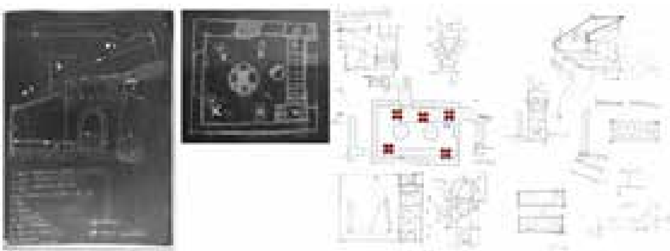
Fig. 148 – Definizione degli eidotipi per il rilievo del complesso del Sepolcro degli Scipioni.
