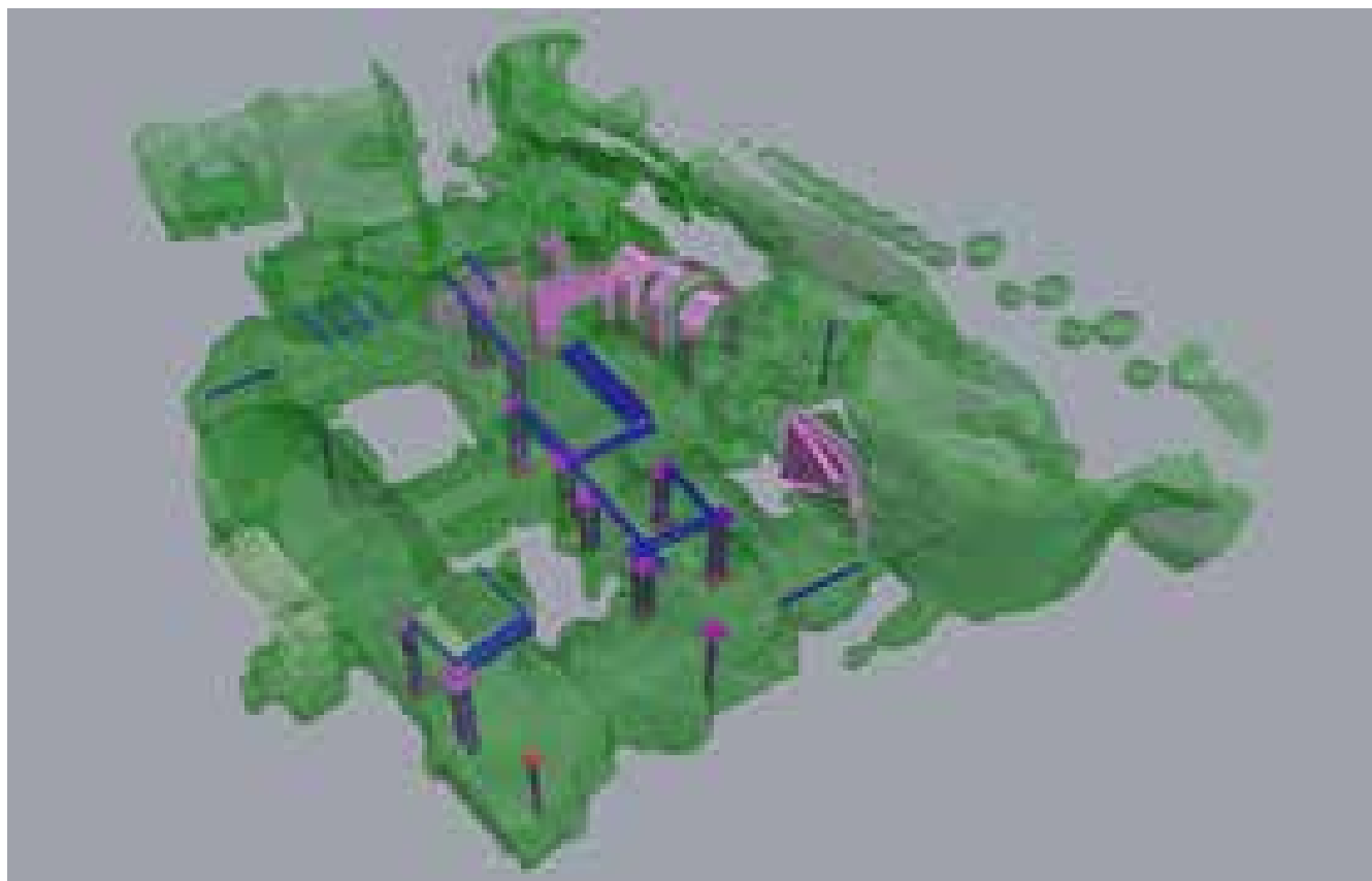
Fig. 174 – Nel caso dei complessi del Sepolcro degli Scipioni, caratterizzato da grande irregolarità delle superfici e da geometrie spesso non riconducibili a forme canoniche, la segmentazione rappresenta una sfida particolarmente complessa.
