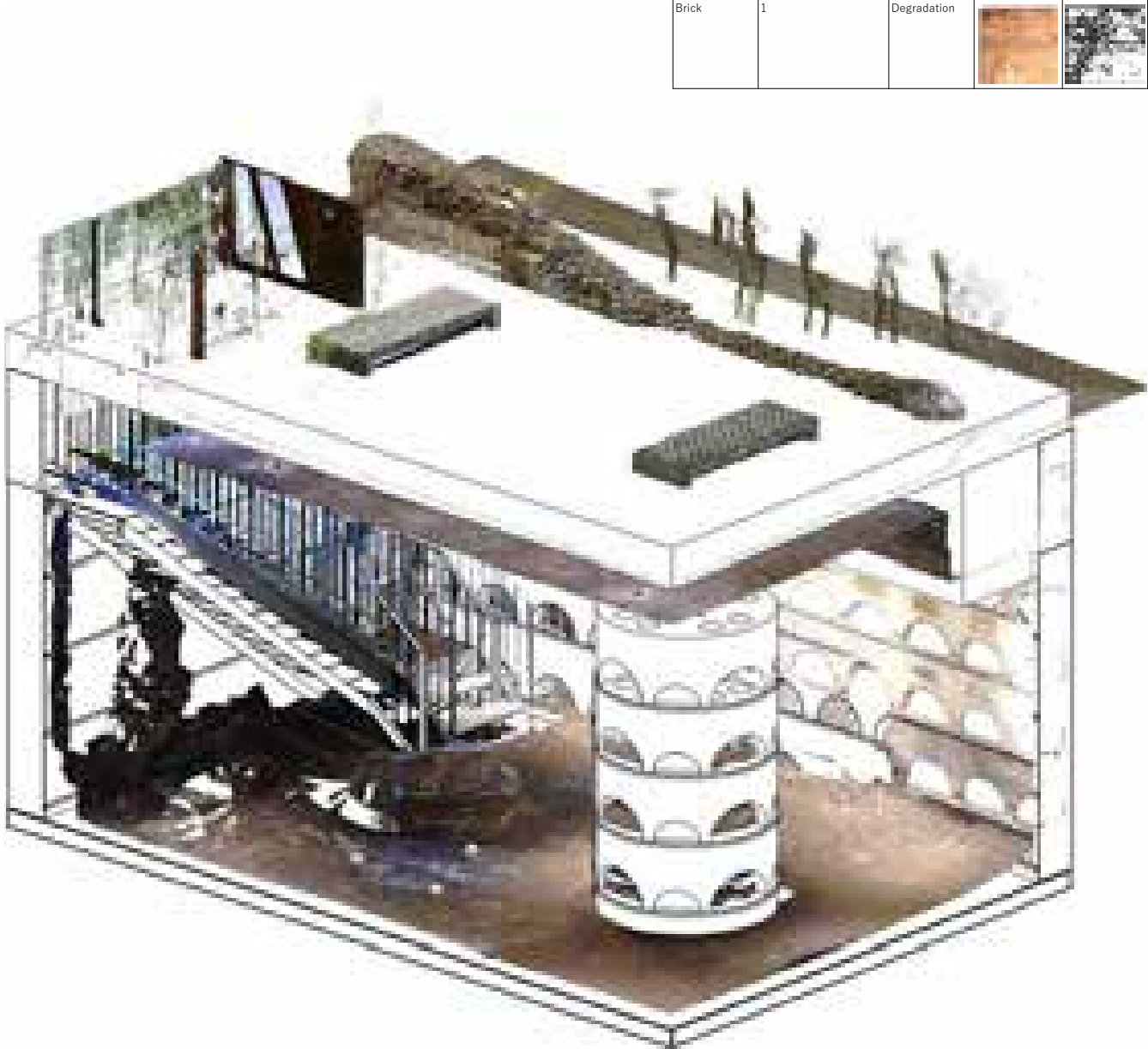
Fig. 23 – Ad ogni componente, dell’oggetto di indagine, sono associate informazioni sul materiale, lo stato di conservazione e il processo di conservazione o restauro. Fig. 23 – Each component of a built heritage asset is associated with information concerning materials, conservation state, and conservation or restoration processes.
