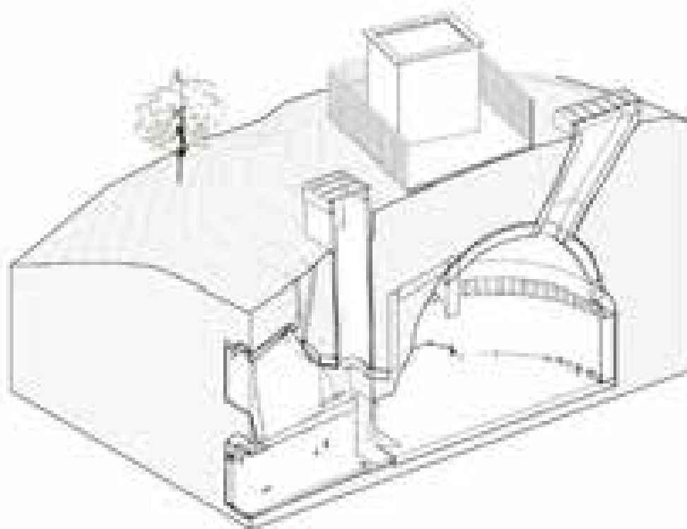
Fig. 21 – I modelli diventano parametrici e sono “informati” con attributi relativi ai materiali, alle tecniche costruttive, allo stato di conservazione e alla cronologia.
