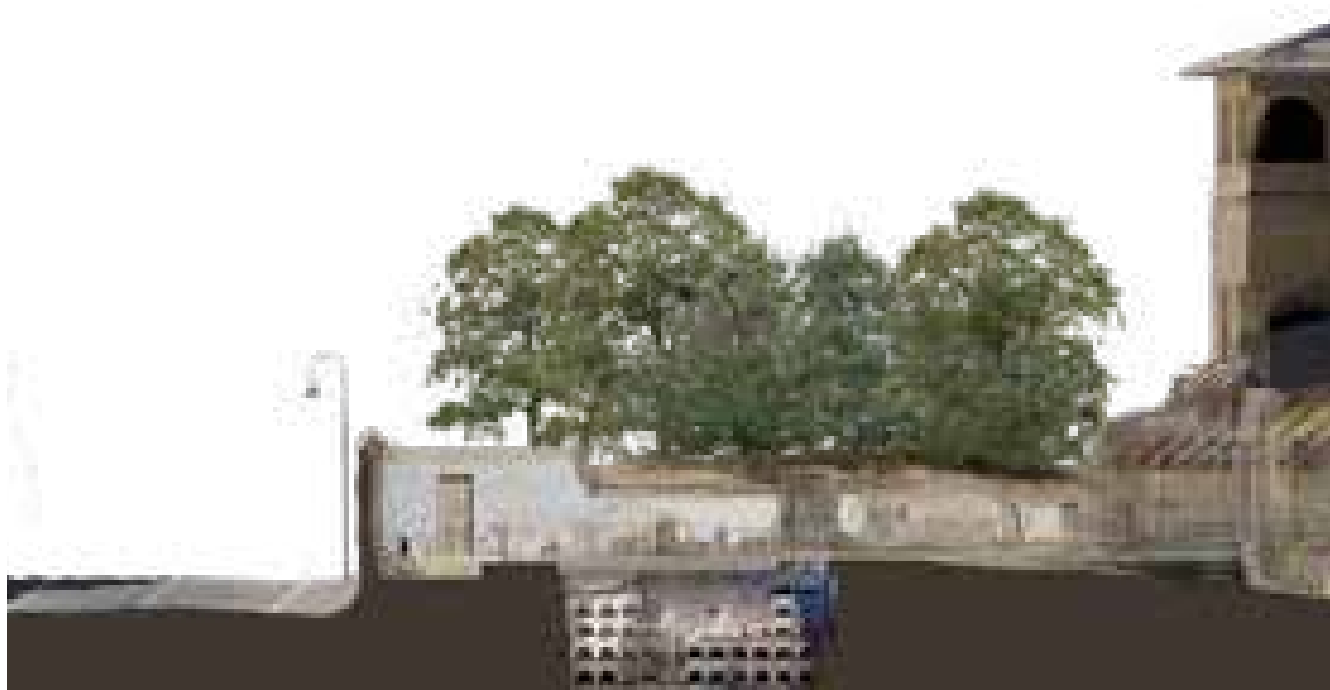
Fig. 188 – Ortofoto che consente di leggere le trasformazioni che nel tempo hanno interessato il complesso del Sepolcro degli Scipioni. Sezione Ovest-Est.
