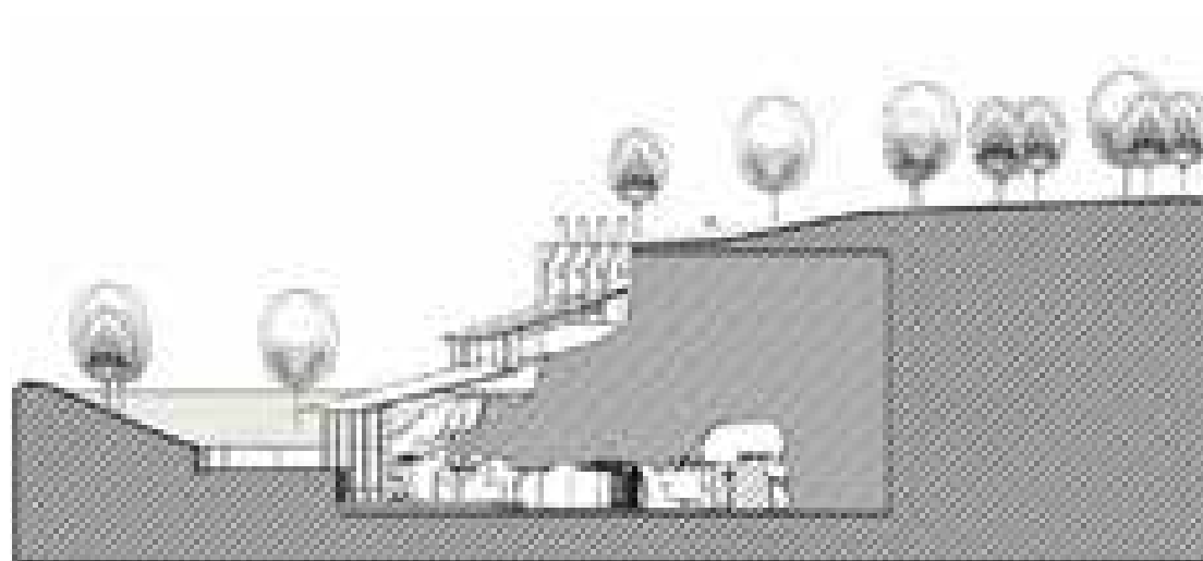
Fig. 226 – Sezione Nord-Sud estratta dal modello informato del complesso del Sepolcro degli Scipioni.
