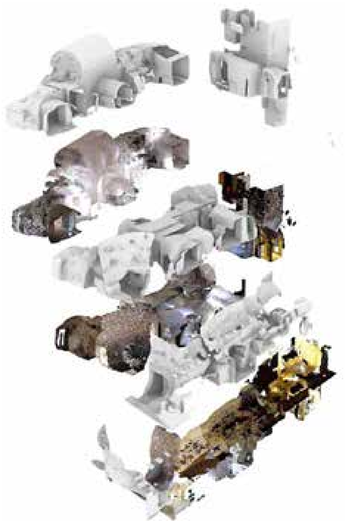
Fig. 173 – Per ciascun elemento architettonico del Sepolcro degli Scipioni è costruito un oggetto parametrico dotato non solo di una forma tridimensionale, ma anche di un insieme articolato di attributi informativi.
