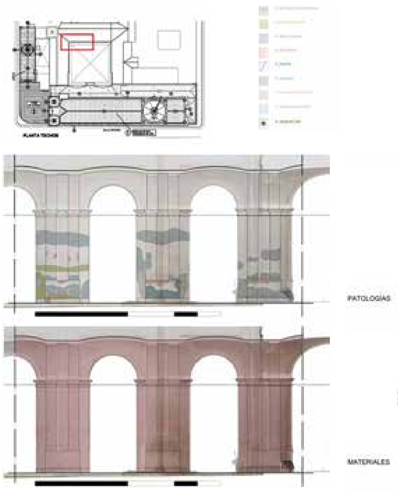
Fig. 99 – Dettaglio della mappatura delle patologie presenti sul lato est della galleria del chiostro (lato esterno).
