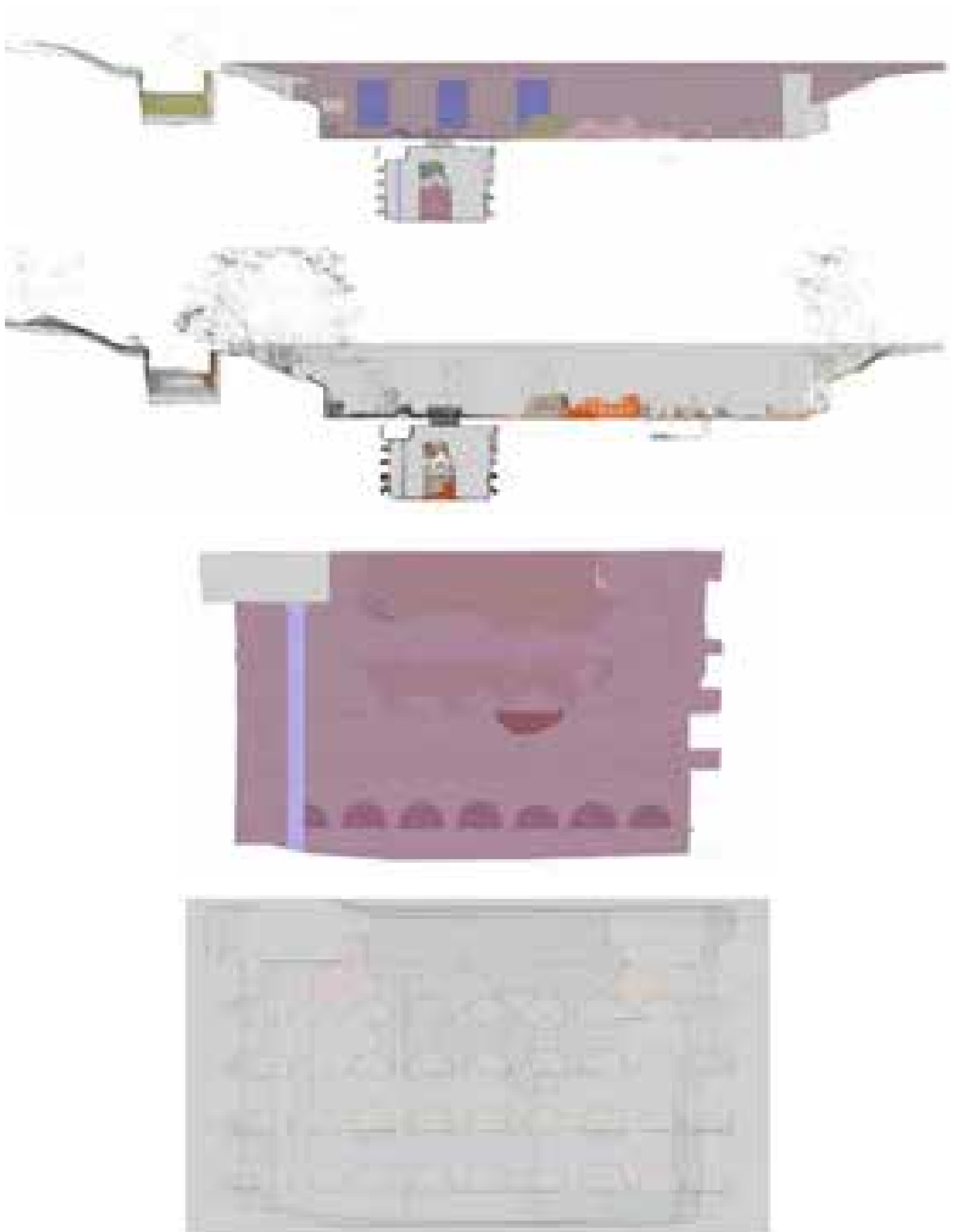
Fig. 210 – Patologie mappate sul modello informato sul Colombario del Sepolcro degli Scipioni. Sezione Sud-Nord.
