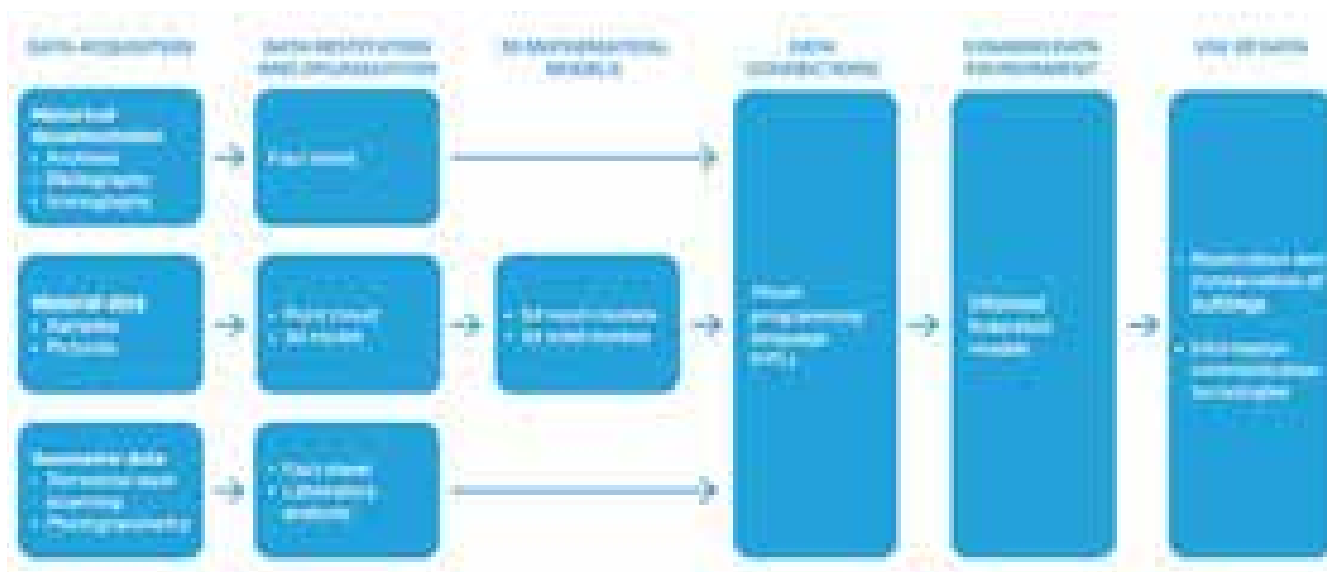
Fig. 8 – Workflow della procedura HBIM applicata.
