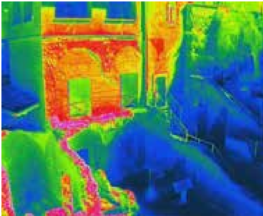
Fig. 170 – Immagine termografica della facciata esterna rivolta a ovest del complesso del Sepolcro degli Scipioni.
