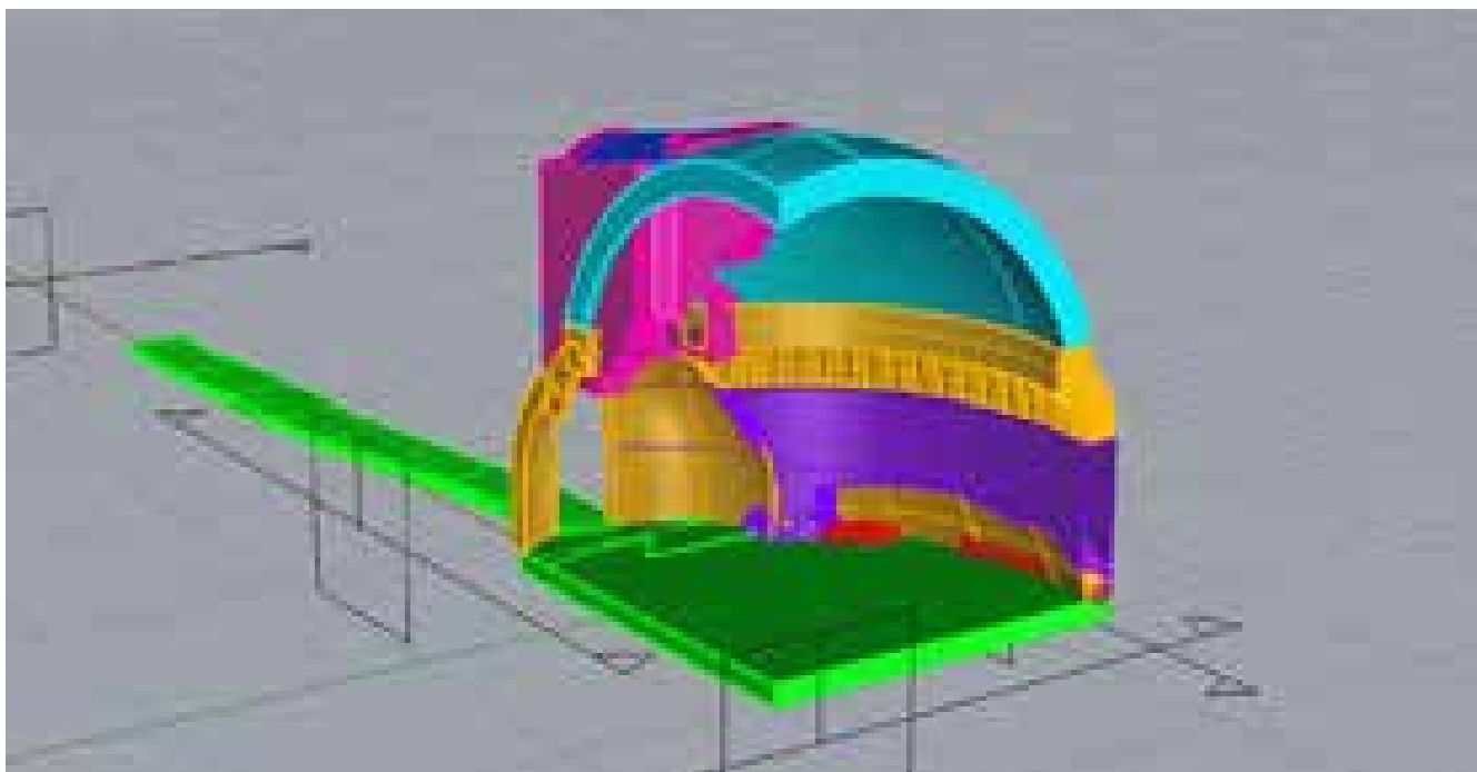
Fig. 176 – Ogni elemento del Mausoleo di Monte del Grano è modellato sulla base della geometria reale, evitando semplificazioni eccessive che potrebbero compromettere la fedeltà del modello.
