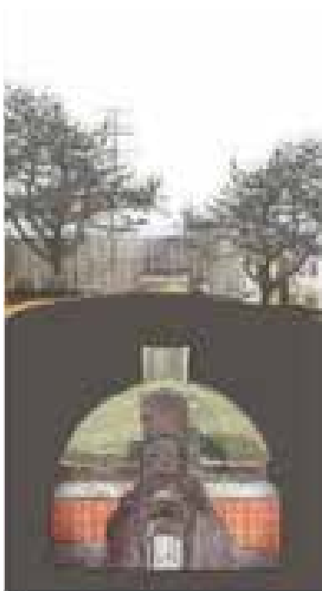
Fig. 205 – Patologie mappate sul modello informato del Mausoleo di Monte del Grano.
