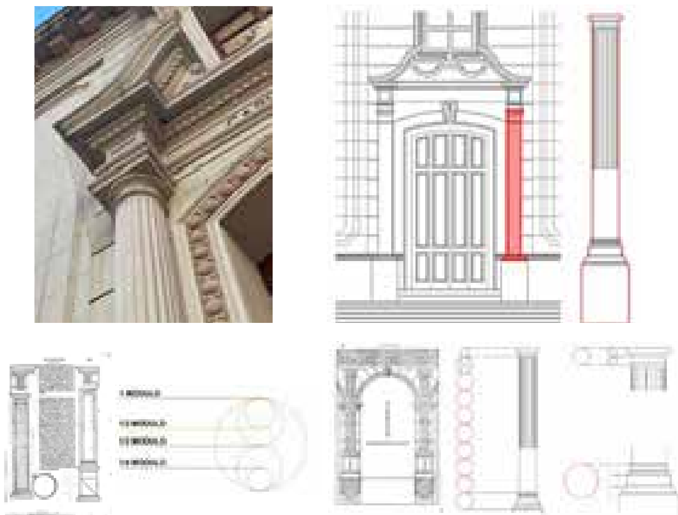
Fig. 78 – Analisi delle proporzioni della facciata della Cappella di San Rocco.
