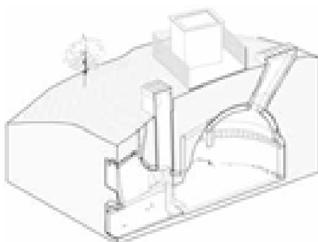
Fig. 221 – Dettaglio dello spaccato longitudinale Ovest-Est della camera sepolcrale e del corridoio d'ingresso estratta dal modello informato del Mausoleo di Monte del Grano.
