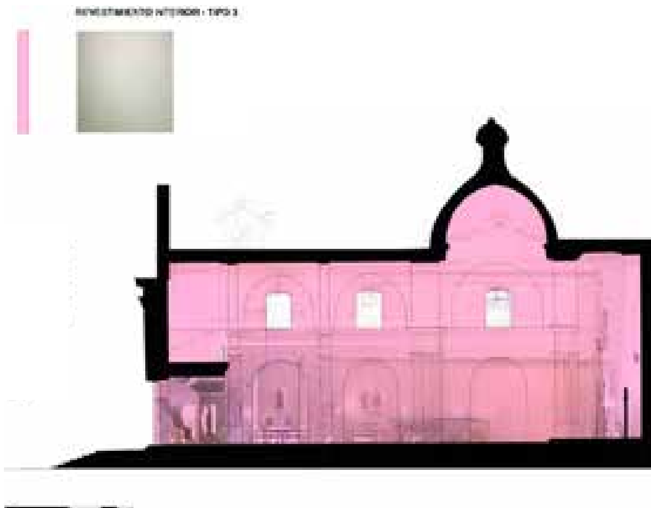
Fig. 72 – Materiali applicati su una sezione della Cappella di San Rocco.
