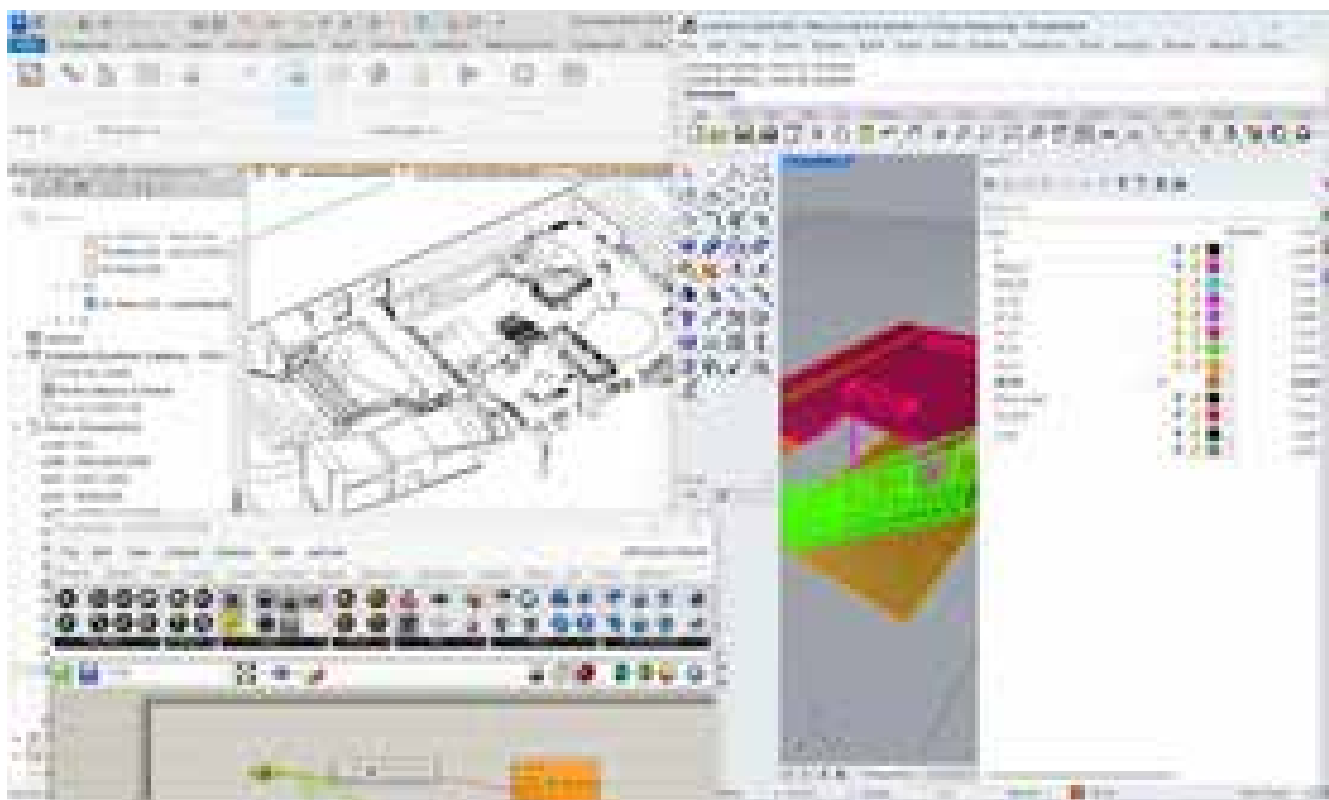
Fig. 194 – Il modello parametrico si trasforma in un archivio diagnostico tridimensionale, nel quale la superficie dell'edificio diventa un'interfaccia interrogabile e non un semplice supporto grafico. Complesso del Sepolcro degli Scipioni.
