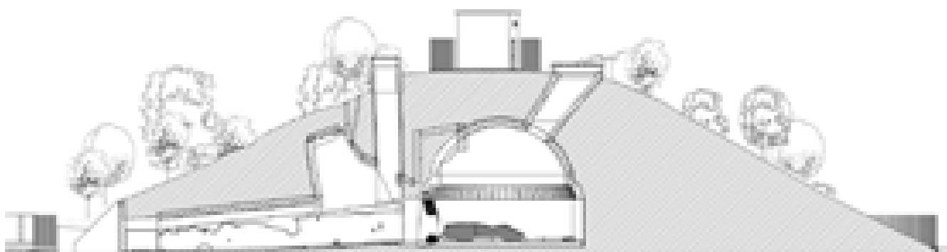
Fig. 217 – Sezione longitudinale Ovest-Est della camera sepolcrale e del corridoio d'ingresso estratta dal modello informato del Mausoleo di Monte del Grano.
