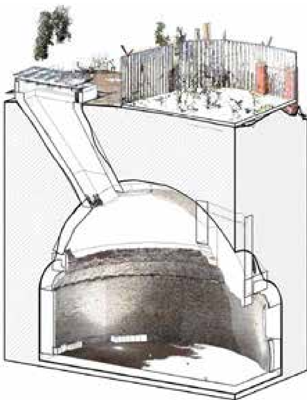
Fig. 203 – Il modello informato Mausoleo di Monte del Grano, permette di mettere in relazione la distribuzione delle efflorescenze saline e delle disgregazioni superficiali con l'andamento delle murature, la presenza di aperture, le zone di contatto con il terreno e le diverse fasi costruttive.
