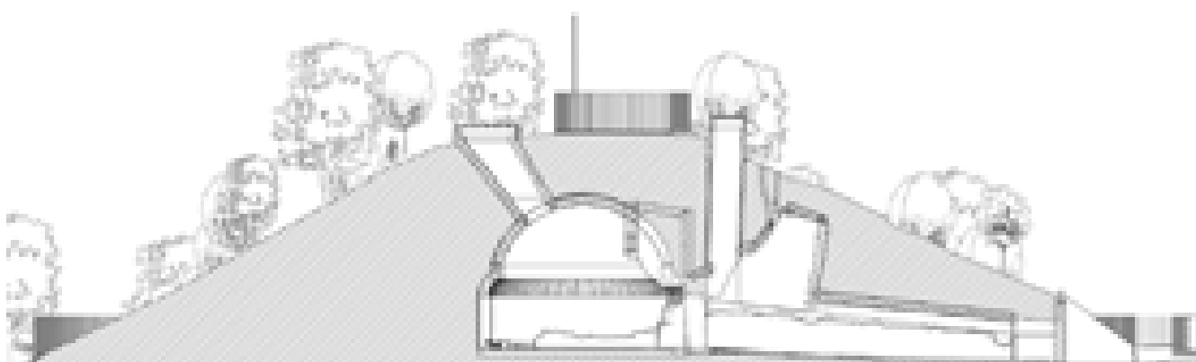
Fig. 218 – Sezione longitudinale Est-Ovest della camera sepolcrale e del corridoio d'ingresso estratta dal modello informato del Mausoleo di Monte del Grano.
