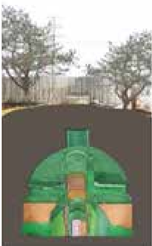
Fig. 196 – Applicazione dei materiali e delle patologie sul modello informato del Mausoleo di Monte del Grano.
