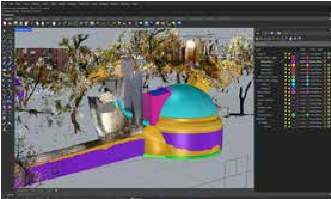
Fig. 18 – Dalla nuvola di punti si sviluppa una modellazione 3D che tiene conto della geometria reale della struttura analizzata.
