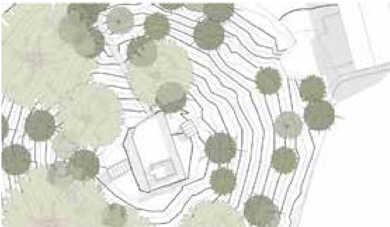
Fig. 214 – Pianta della parte superiore del mausoleo estratta dal modello informato del Mausoleo di Monte del Grano.
