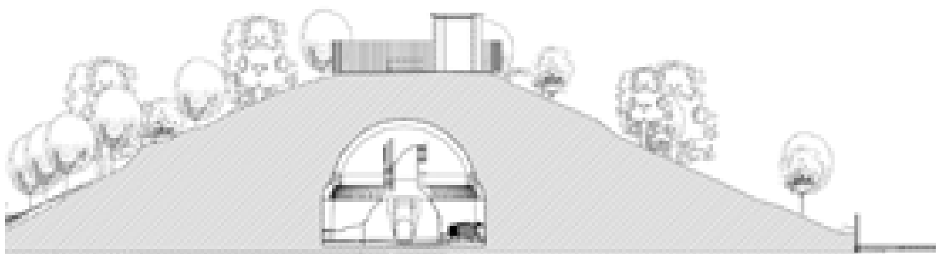
Fig. 219 – Sezione trasversale della camera sepolcrale sulla parte del corridoio estratta dal modello informato del Mausoleo di Monte del Grano.
