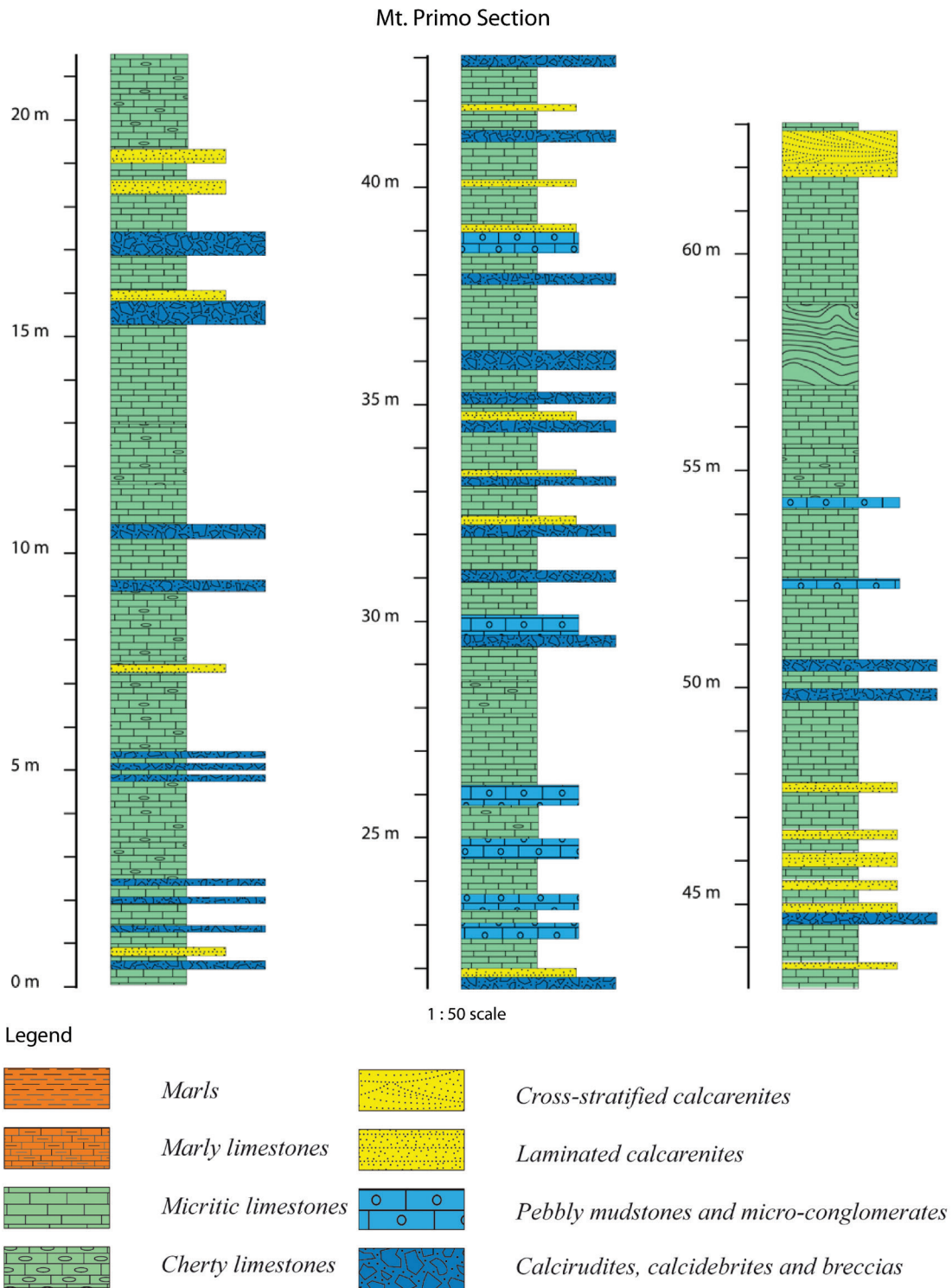
Fig. 9 - The Mt. Primo section stratigraphic log.
